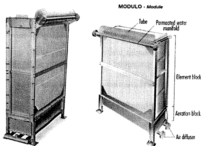
Figura 2: Rappresentazione grafica di un modulo MBTR modello TORAY - Everblue o similari
