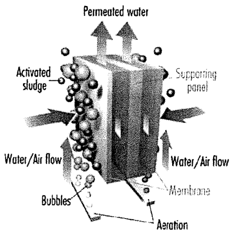
Figura 1: Particolare costruttivo delle membrane MBR e schema di funzionamento
