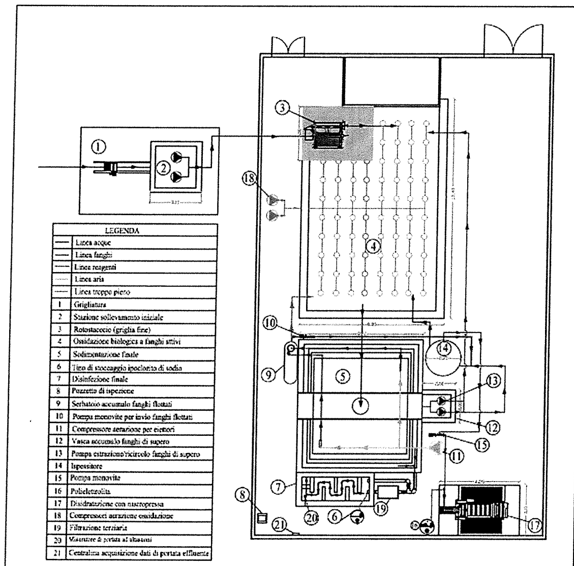
Figura 3: Stato di fatto dello schema dell'impianto di depurazione
