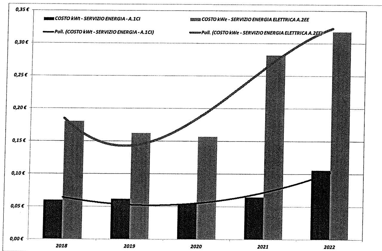
GRAFICO 2 – COSTO MEDI DEL VETTORE ENERGETICO NEL PERIODO DI VIGENZA DEL CONTRATTO MIES2
